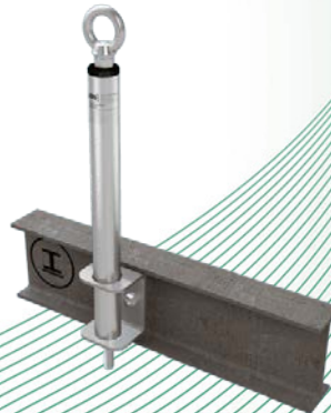
Bild 14: ABS-Lock® III-SEITL-SR (Montagebeispiel an Stahl)
