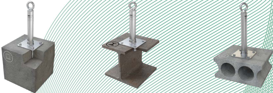
Bilder 1 - 3: Anschlageinrichtung, Typ: ABS-Lock® X-SR mit Hülse (Montagebeispiele)
