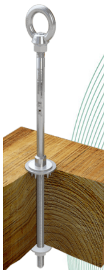
Bild 1: Anschlageinrichtung, Typ: ABS-Lock® III
