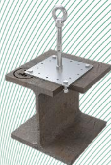
Bild 7: Anschlagseinrichtung, Typ: ABS-Lock® X-ST
