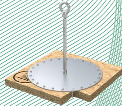
Bild 14: Anschlageinrichtung, Typ: ABS-Lock® X-H-24
