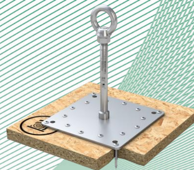
Bild 8: Anschlagseinrichtung, Typ: ABS-Lock® X-H-16
