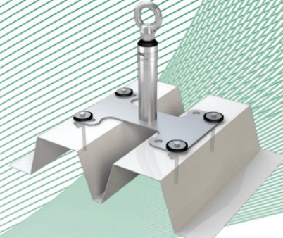
Bild 16: Anschlageinrichtung, Typ: ABS-Lock® X-T-21
