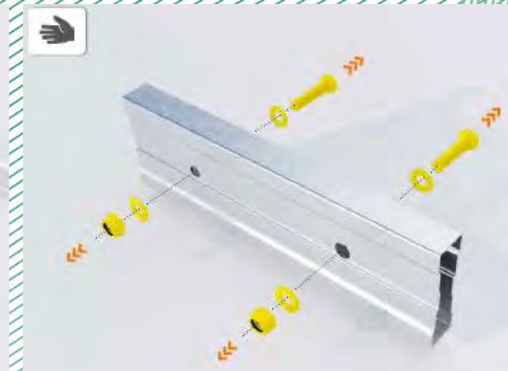
Bild 3: Leiterverbinder
