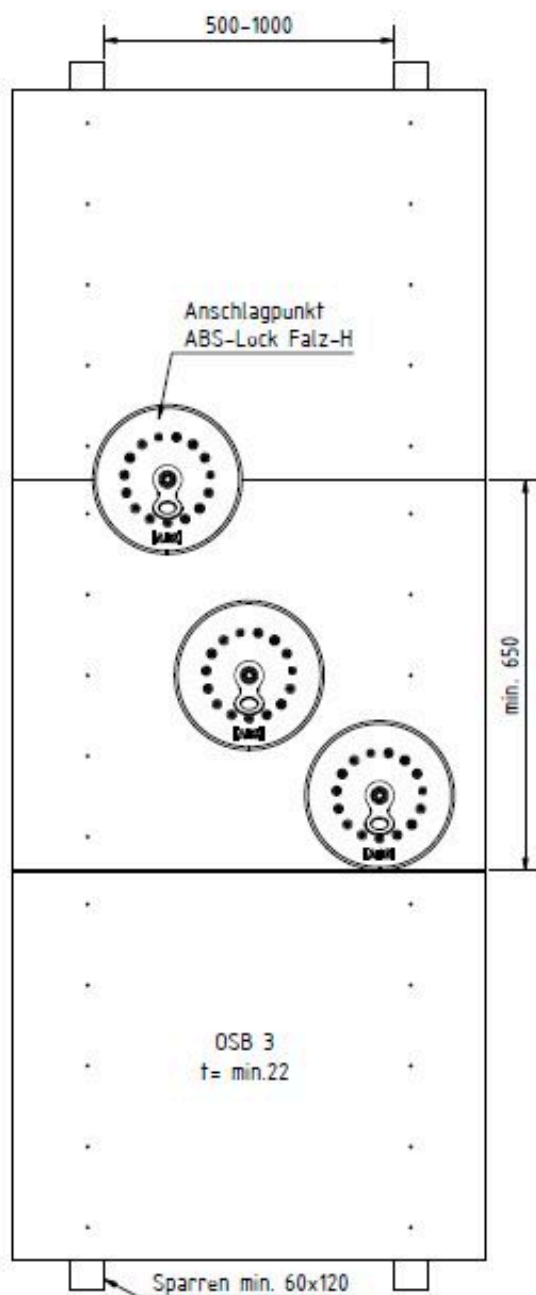
Abbildung 3 - Aufbauvariante OSB3 [Maße in mm]
